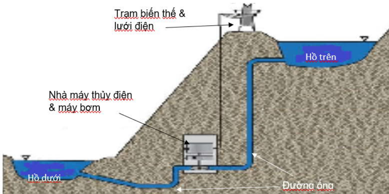
Lược đồ các hạng mục nhà máy thủy điện tích năng
