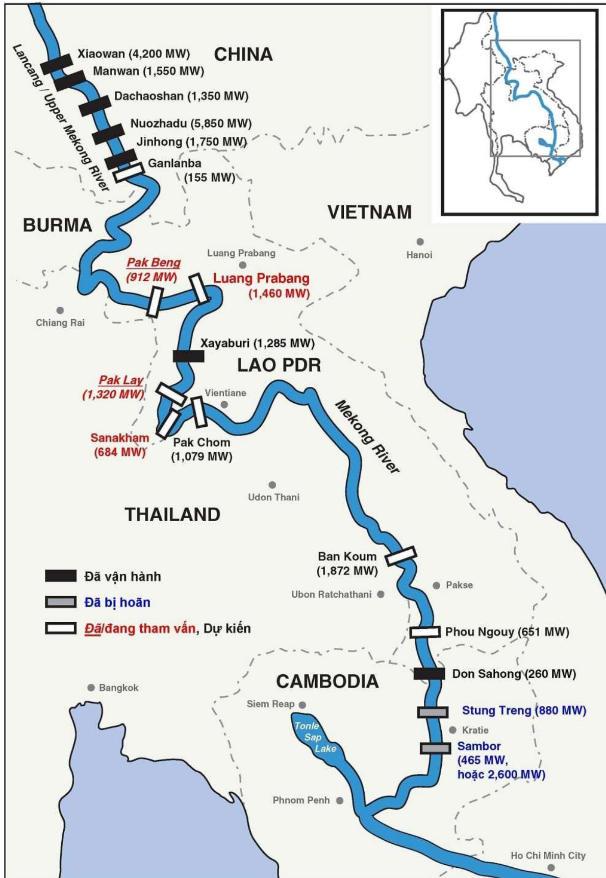
Vị trí, hiện trạng và công suất các dự án thủy điện trên dòng chính Mekong đến tháng 5.2019.
