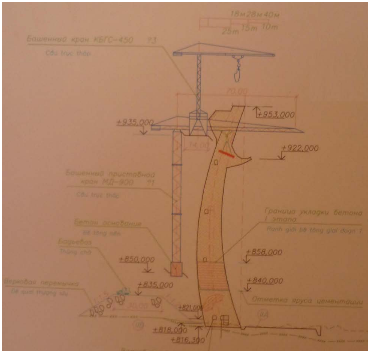
Mặt cắt ngang đập và cần trục thi công
