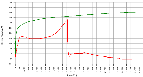
Hình 20. Diễn biến ứng suất trên mặt dờng thi công ở cao độ 122.00 m
