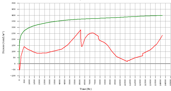
Hình 18. Diễn biến ứng suất trên biên thượng lưu cao độ 107.83m
