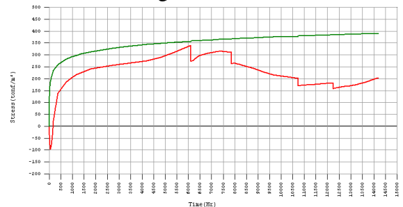
Hình 17. Diễn biến ứng suất trên đỉnh hành lang cao độ 105.00m
