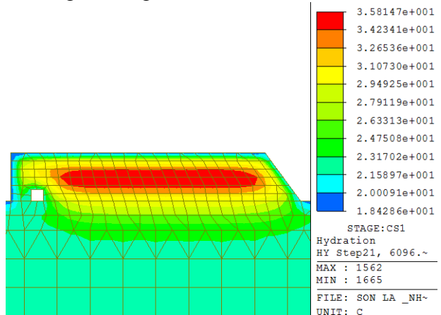
Hình 10. Phân bố nhiệt độ thân đập ở 6096 (h)
