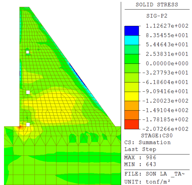
Hình 16. Trường ứng suất ở 14208 giờ
