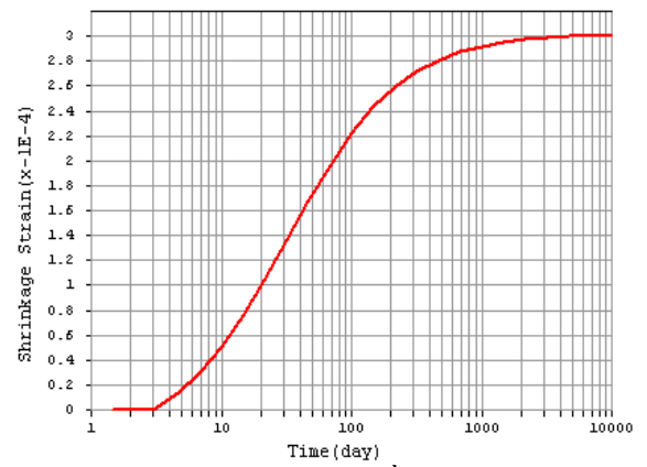
Hình 6. Co ngót của bê tông đầm lẫn theo thời gian
