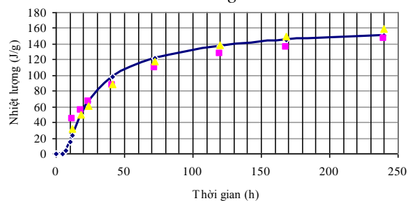
Hình 3. Đường cong nhiệt thủy hoá của bê tông đầm lăn theo thời gian
