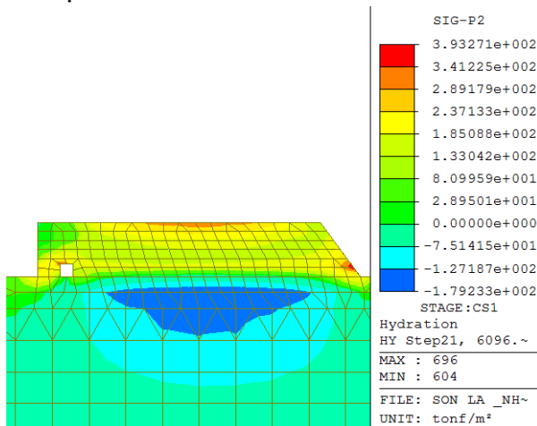
Hình 15. Trường ứng suất ở 6096 giờ
