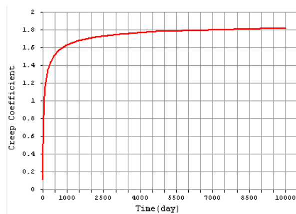
Hình 5. Từ biến của bê tông đầm lẫn theo thời gian
