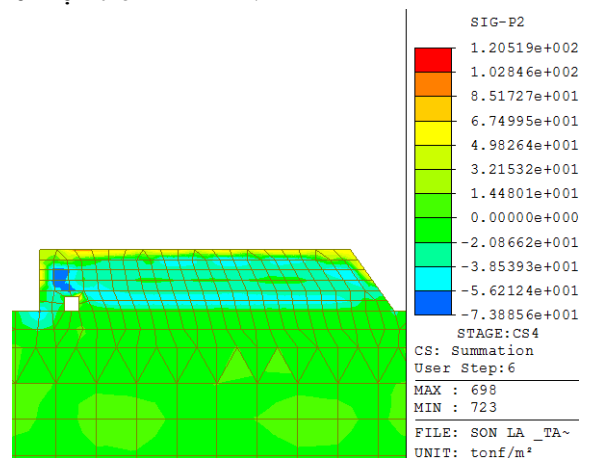
Hình 14. Trường ứng suất ở 1368 giờ
