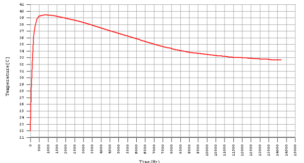
Hình 13. Diễn biến nhiệt độ lõi đập cao độ 113.5m
