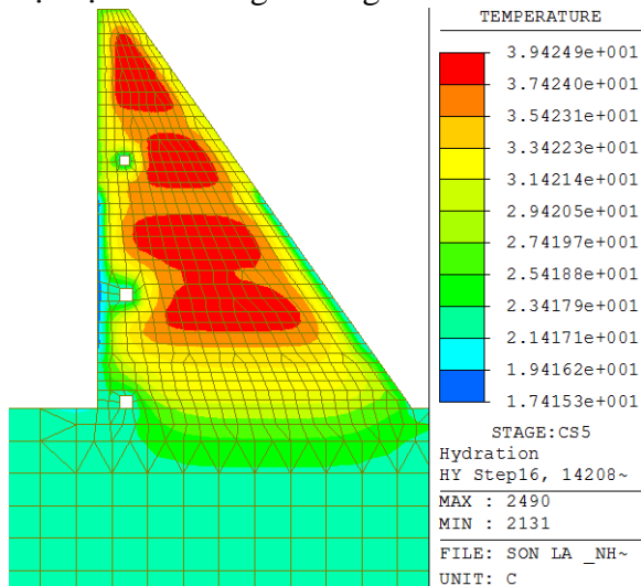
Hình 11. Phân bố nhiệt độ thân đập ở 14208 (h)
