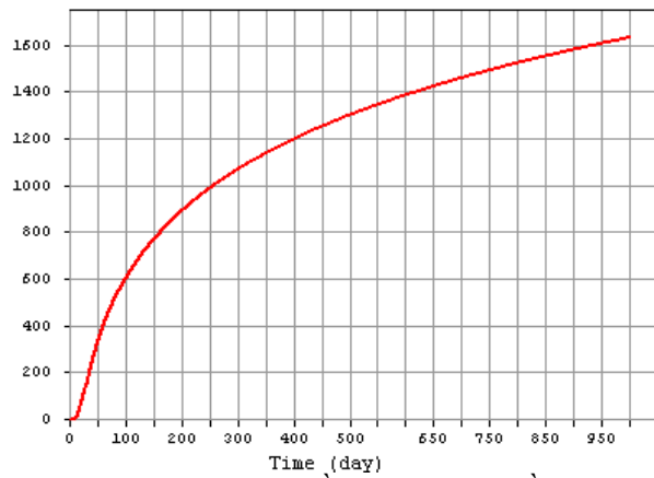
Hình 4. Môđun đàn hồi của bê tông đầm theo thời gian
