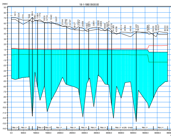
Hình 17: Mực nước dọc sông Trà Lý (Trường hợp xây dựng 2 đập ở đầu và cuối sông Trà Lý)
