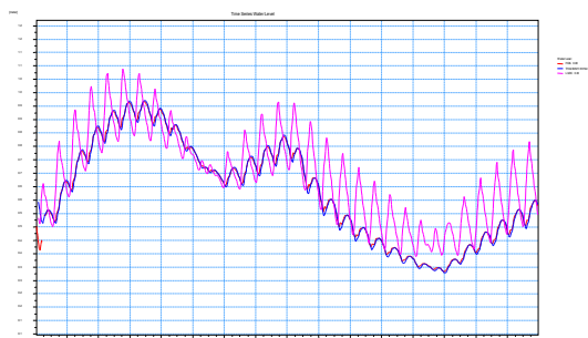
Hình 14: Quá trình mực nước tại ngã ba Hóa-Luộc, ngã ba Thái Bình-Luộc và ngã ba Hồng-Luộc (Trường hợp xây dựng đập trên sông Hoá, Thái Bình, Mới)
