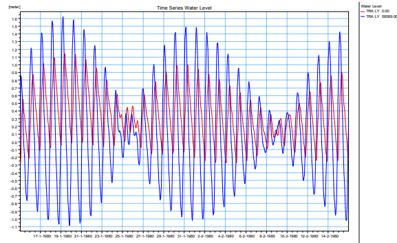
Hình 6: Đường mực nước tại ngã ba Hồng-Trà Lý và cuối Trà Lý – PA0
