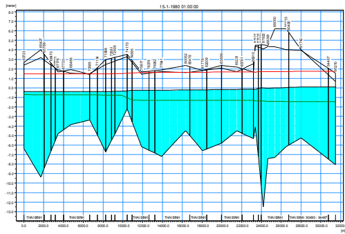
Hình 3: Mực nước dọc sông Thái Bình – PA0
