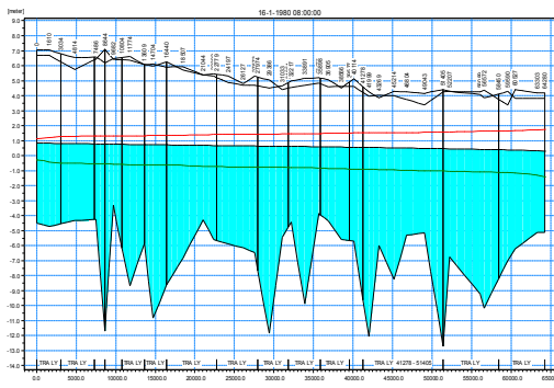
Hình 5: Mực nước dọc sông Trà Lý – PA0
