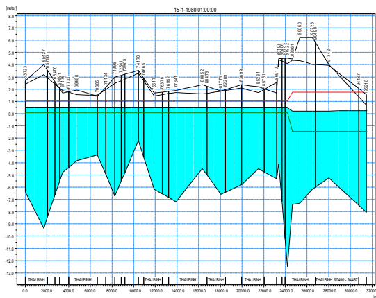
Hình 12: Mực nước dọc sông Thái Bình (Trường hợp xây dựng đập trên sông Hoá, Thái Bình, Mới)
