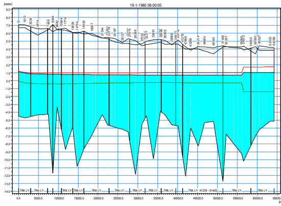
Hình 15: Mực nước dọc sông Trà Lý (Trường hợp xây dựng 1 đập ở cuối sông Trà Lý)
