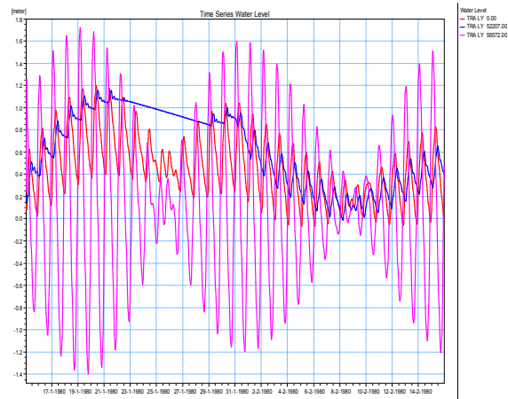
Hình 18: Quá trình mực nước tại ngã ba Hồng-Trà Lý, thượng và hạ lưu đập Trà Lý (Trường hợp xây dựng 2 đập ở đầu và cuối sông Trà Lý)
