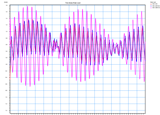
Hình 9: Đường quá trình mực nước tại ngã ba Hóa-Luộc, thượng lưu và hạ lưu đập sông Hóa (Trường hợp xây dựng 1 đập ở cuối sông Hoá)
