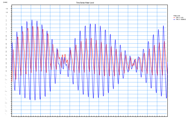
Hình 16: Quá trình mực nước tại ngã ba Hồng-Trà Lý, hạ lưu đập Trà Lý (Trường hợp xây dựng 1 đập ở cuối sông Trà Lý)
