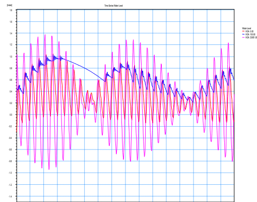
Hình 11: Đường quá trình mực nước tại ngã ba Hóa-Luộc, thượng lưu và hạ lưu đập sông Hóa (Trường hợp xây dựng 2 đập trên sông Hoá)
