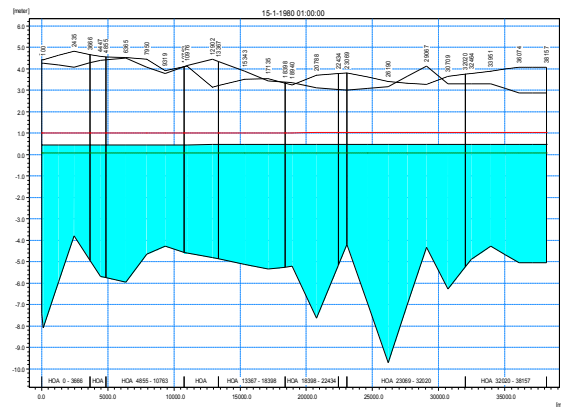
Hình 13: Mực nước dọc sông Hóa (Trường hợp xây dựng đập trên sông Hoá, Thái Bình, Mới)
